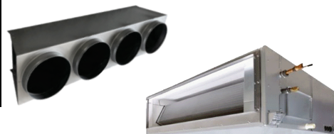
RAV – RM 2241/2801 DTP – E2 MMD – UP 0721/0961 HP – E1 (DRV) HAUTE PRESSION
