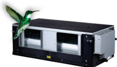
AF-DH 140 et 160 - 1 (~2200 et 2600m3/h)
