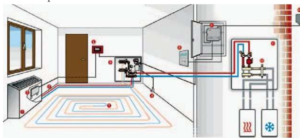
Raccordement d'une installation : Pompe à chaleur / Ventilateur-convecteur Pompe à chaleur / Plancher chauffant rafraîchissant
