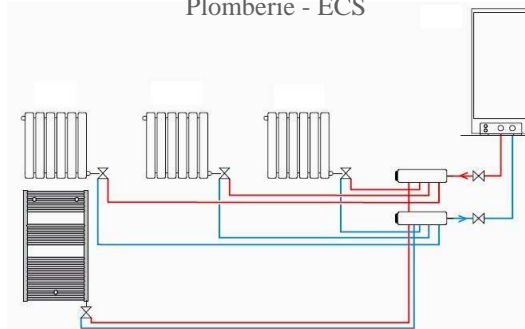
Raccordement d'une installation : Chaudière / Radiateur basse ou haute température Plomberie - ECS
