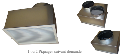
1 ou 2 Piquages suivant demande
